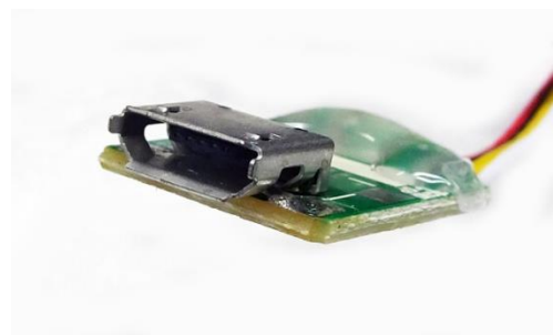
USB ポート拡大写真 (Micro-B)
