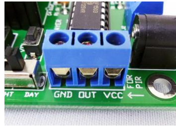
<基板のターミナル(J3)写真>
