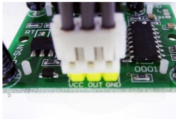
＜PIRセンサーの裏面写真＞
