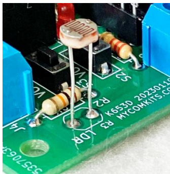
←LDRを浮かしてハンダ付け
