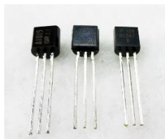
←左から2SA1015、BC557、BC547
