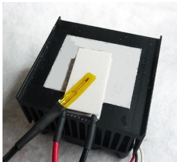
←取り付け例
