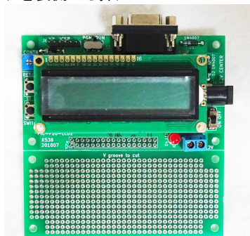
液晶表示パネルにピンヘッダを裏側から挿入
